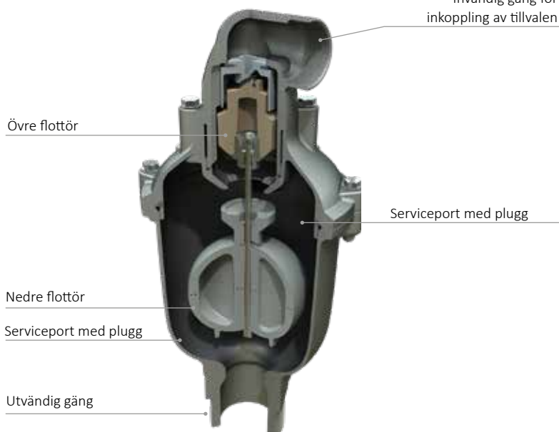
Tryckutjämningsventil (C30-50-SP)
