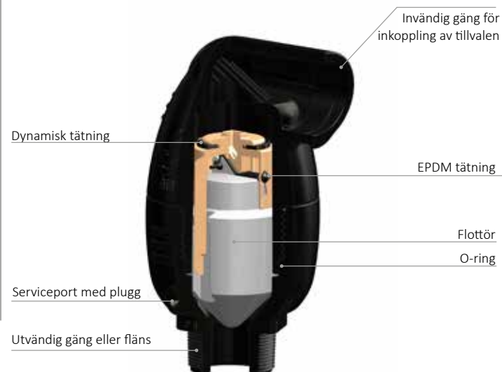
Snorkel SSN-luft
